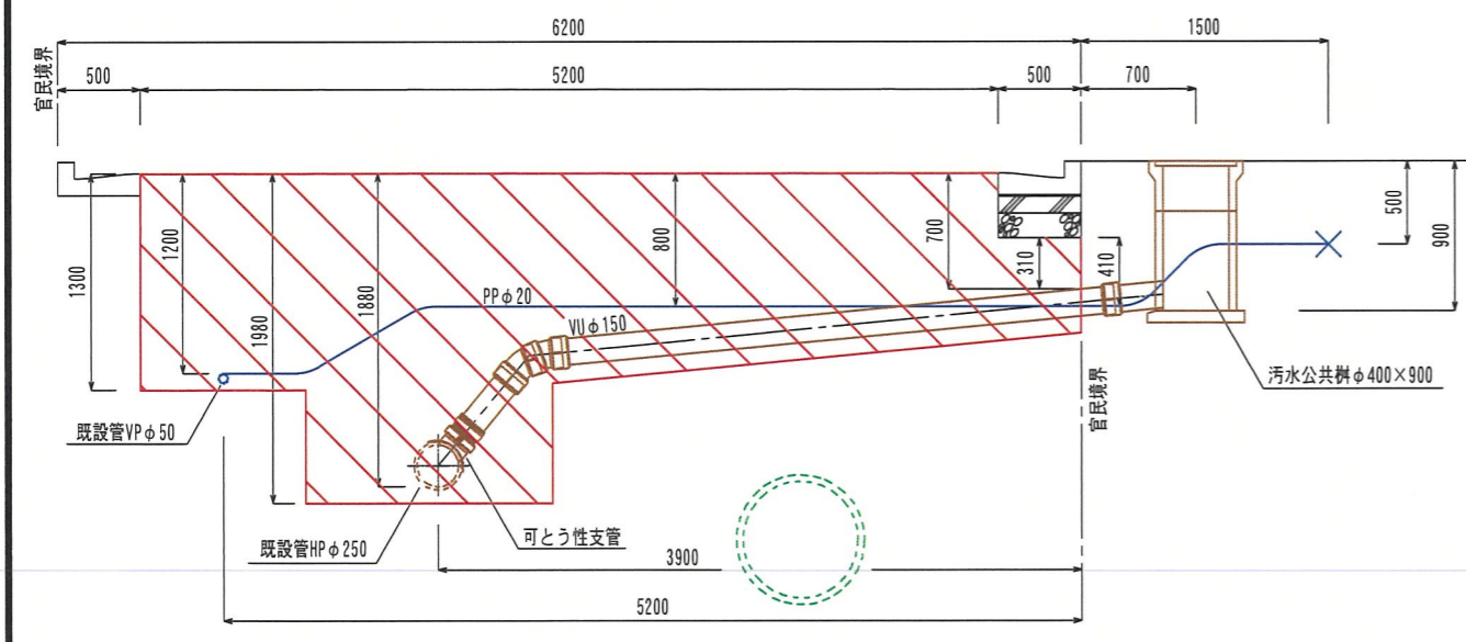
断面図 S=1:50 土留施工 (給水管・汚水管取出し)
