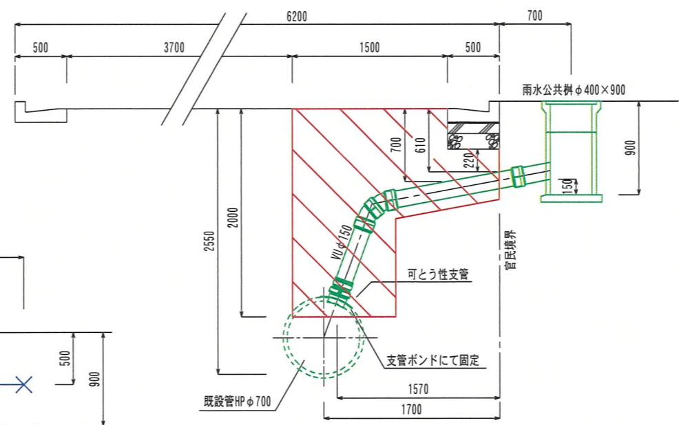
断面図 S=1:50 土留施工 (雨水管取出し)
