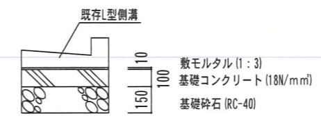
L型側溝復旧断面図
